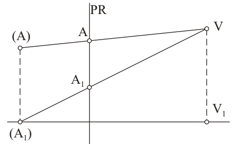
proxeccións dun punto do espacio real no Plano da Representación
