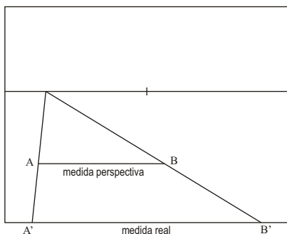
Segmento paralelo a LT en PH
