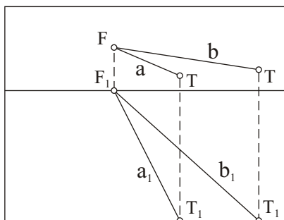
Paralelismo entre rectas
