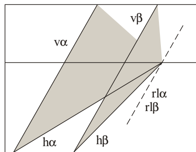
Paralelismo entre planos
