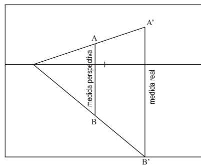
Segmento vertical a partir de PH
